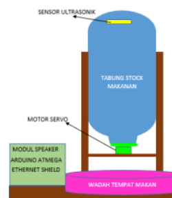
Gambar 6. Rancangan Mekanik Alat Otomatis
