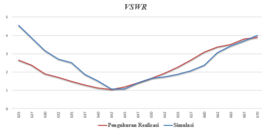
Gambar 5 Grafik VSWR hasil pengukuran realisasi dan simulasi
