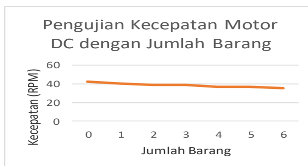
Gambar 3. Grafik Pengujian Kecepatan Motor DC
