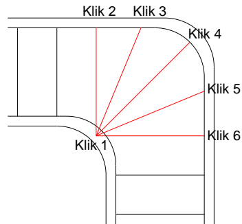
Gambar 4.4 Penggunaan perintah RAY dalam menggambar denah tangga
