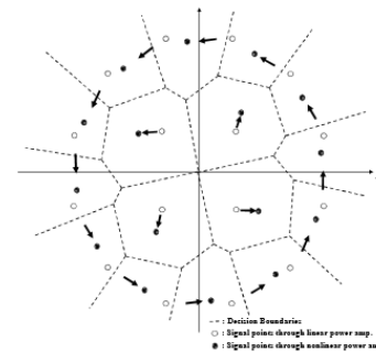
Gambar 2. 4+12 APSK Konstelasi
